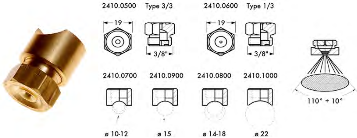
Wassersprühdüsen / Water Spray Nozzle 3/8"
