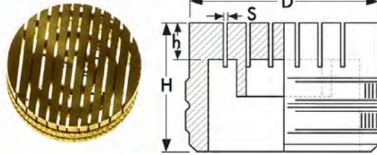
Messing-Schlitzdüse
