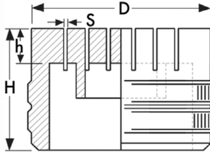
Aluminium Schlitzdüse
