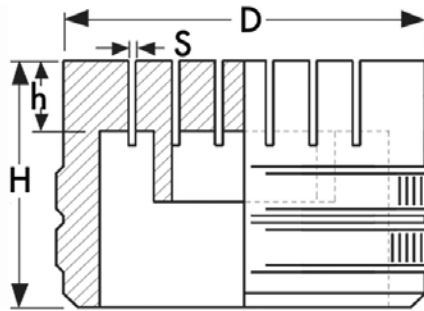
Aluminium Schlitzdüse
