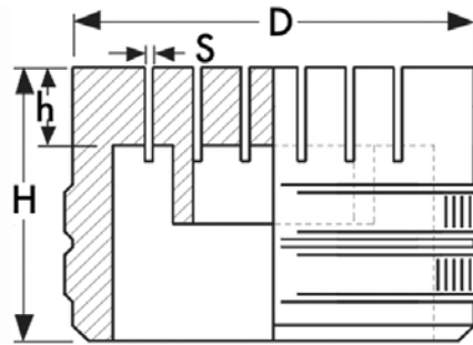
Aluminium Schlitzdüse
