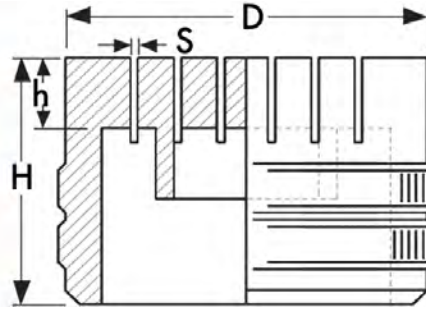
Messing-Schlitzdüse
