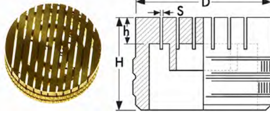
Messing-Schlitzdüse
