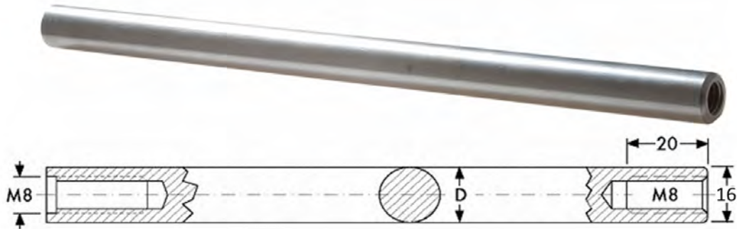
Auswerferstangen / Ejector rods 16 mm
