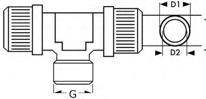
T- Verschraubung
