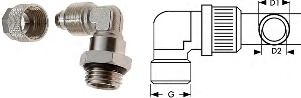
Winkelverschraubung
