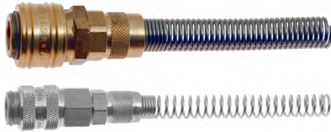
Schnellschlusskupplung 80.03.00.30
